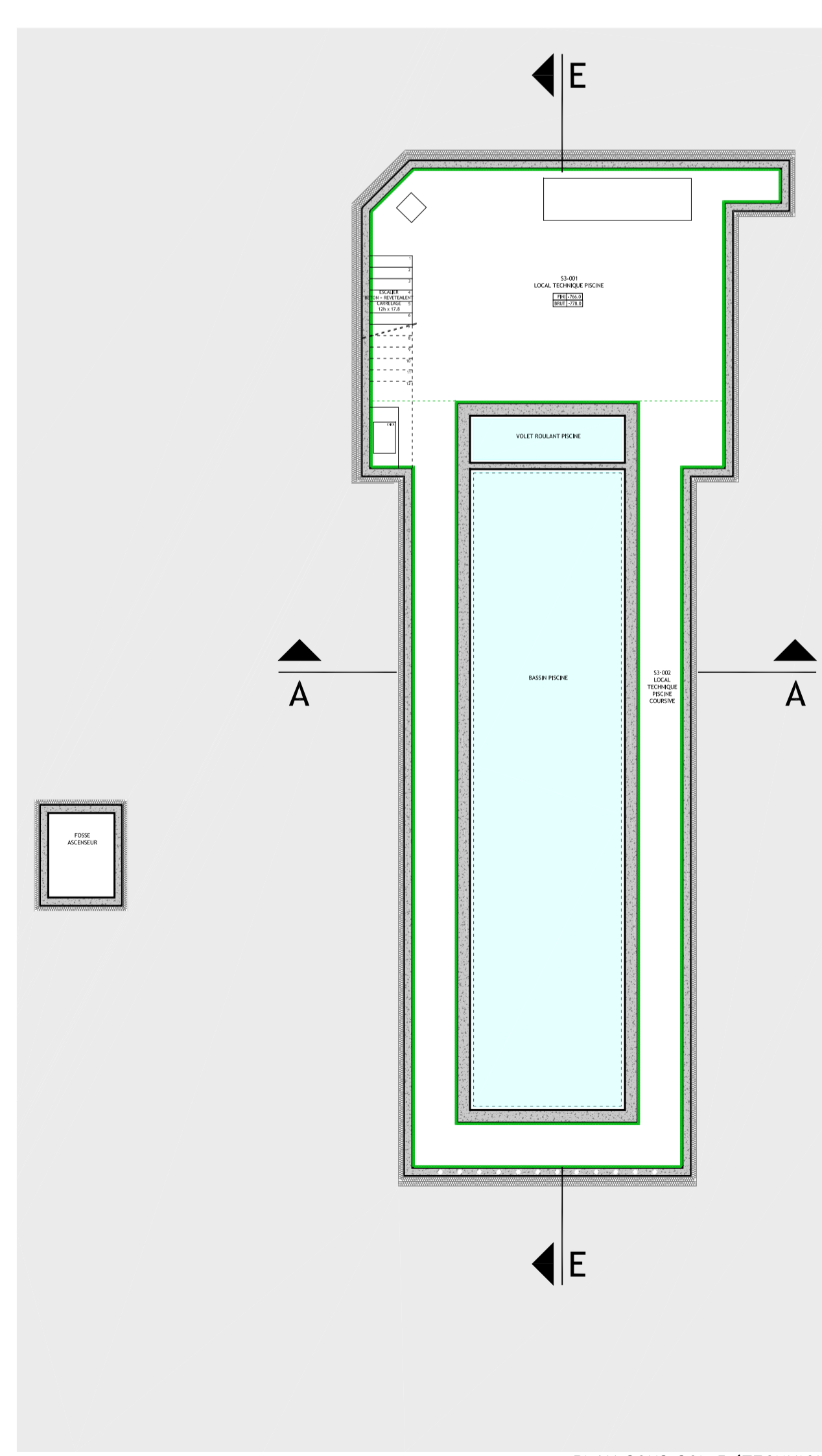
PLAN SOUS SOL 3 (TECHNIQUE)
