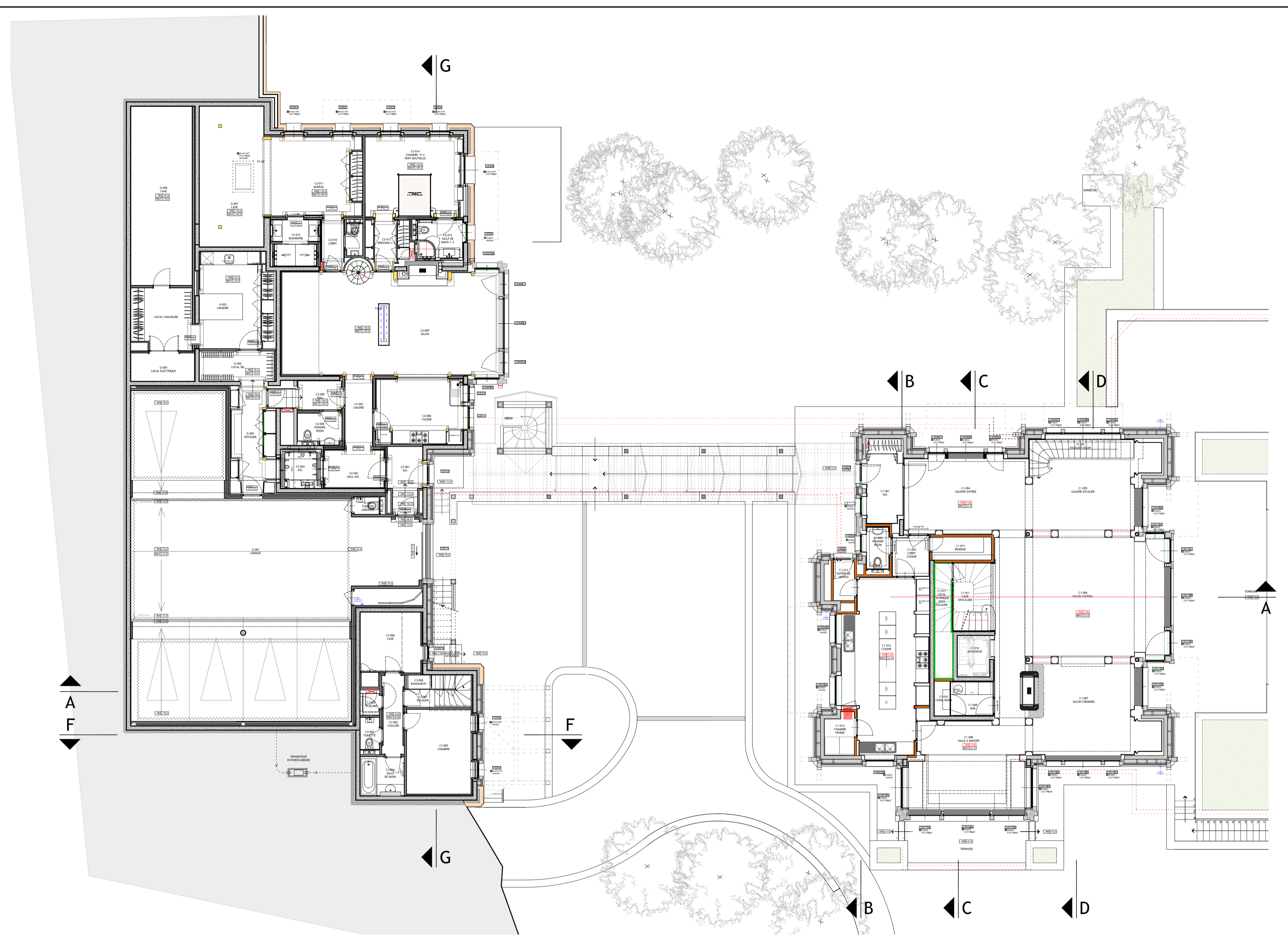
PLAN DU REZ DE CHAUSSEE
