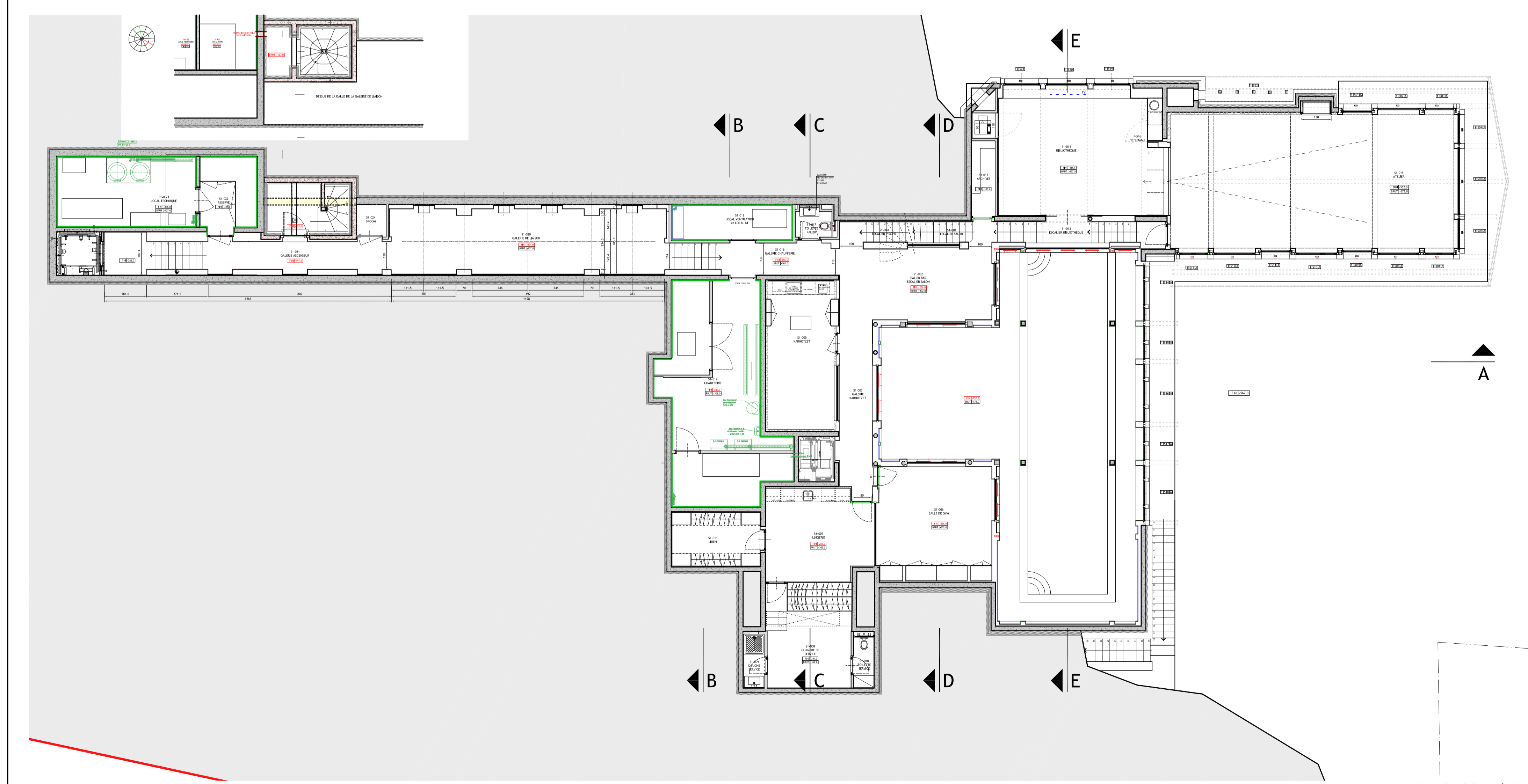
PLAN SOUS SOL 1 (BIBLIO)
