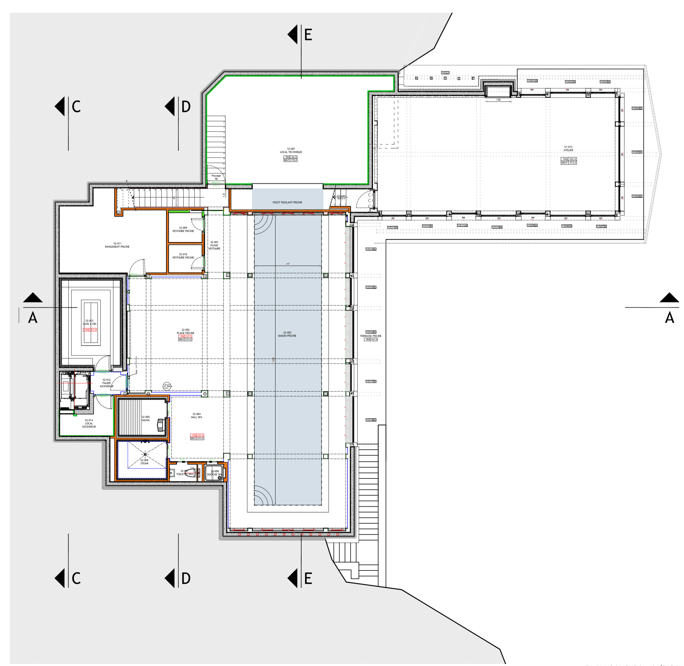
PLAN SOUS SOL 2 (PISCINE)
