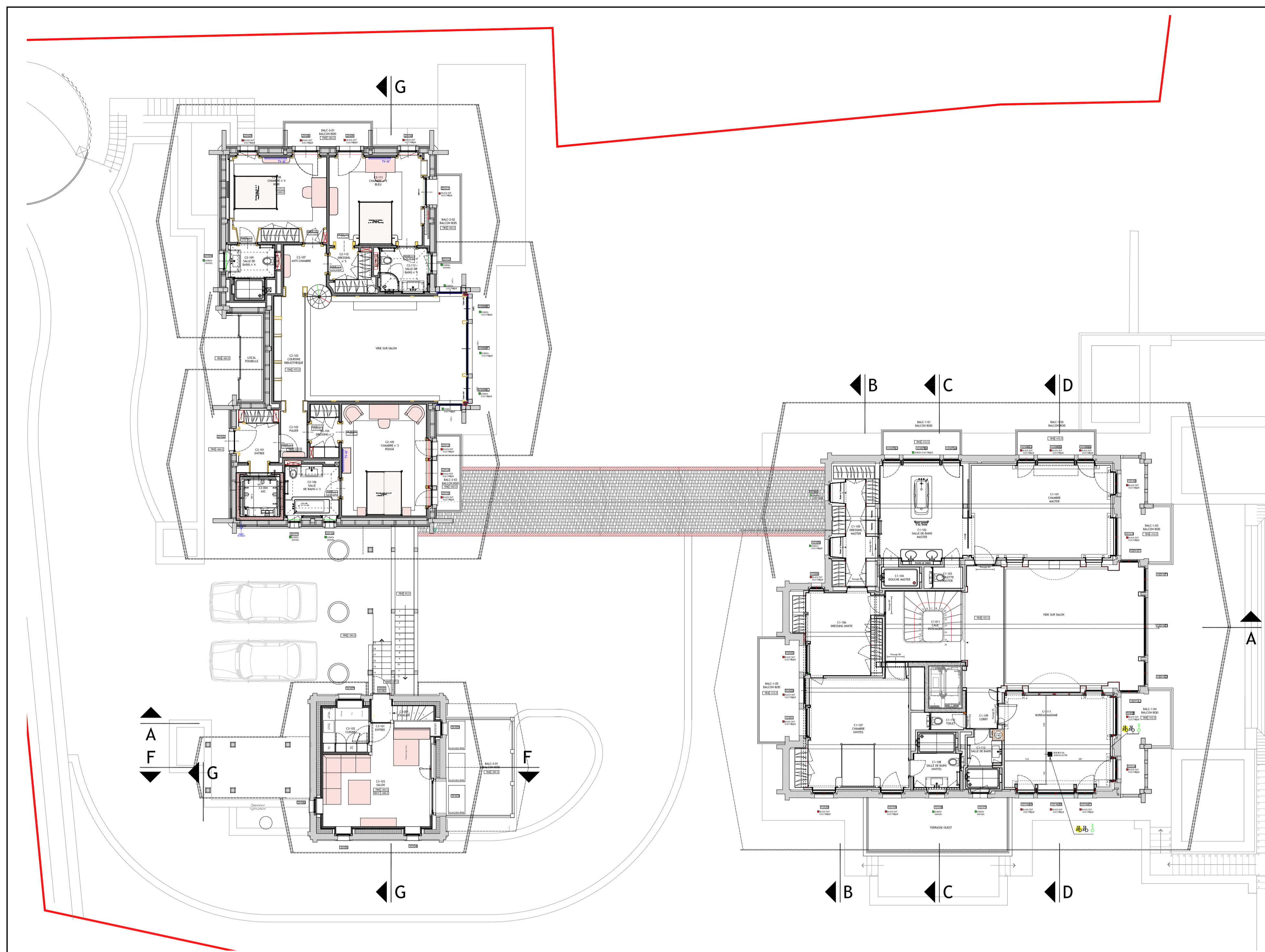
PLAN DU 1ER ETAGE
